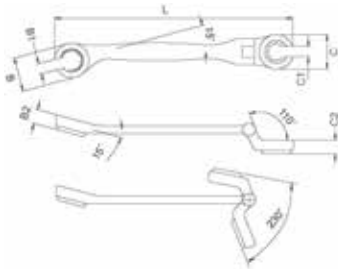
Offener Doppelringschlüssel mit Doppelgelenk
